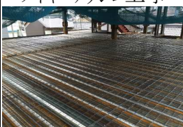
ワイヤーメッシュ工事
