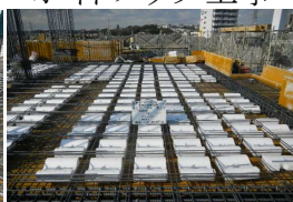
ボイドスラブ工事
